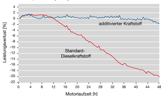
CEC DW-10 Injektorablagerungstest mit B10 Dieselmotorenkraftstoff in PKW Motor
